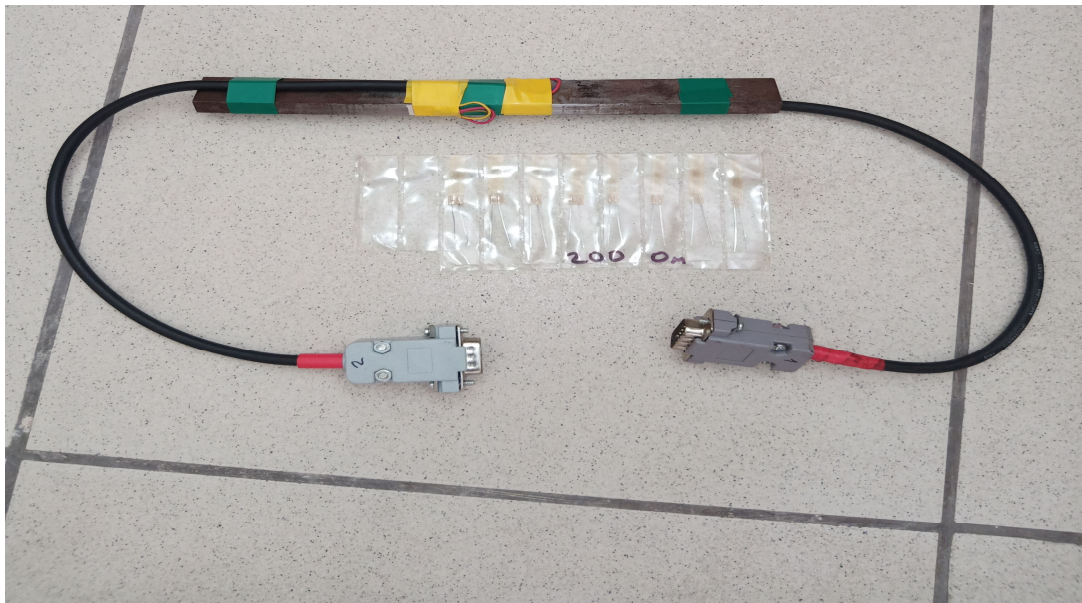
Тарування тензорезисторів з допомогою призматичної балки
